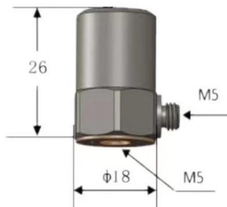
外形示意图
